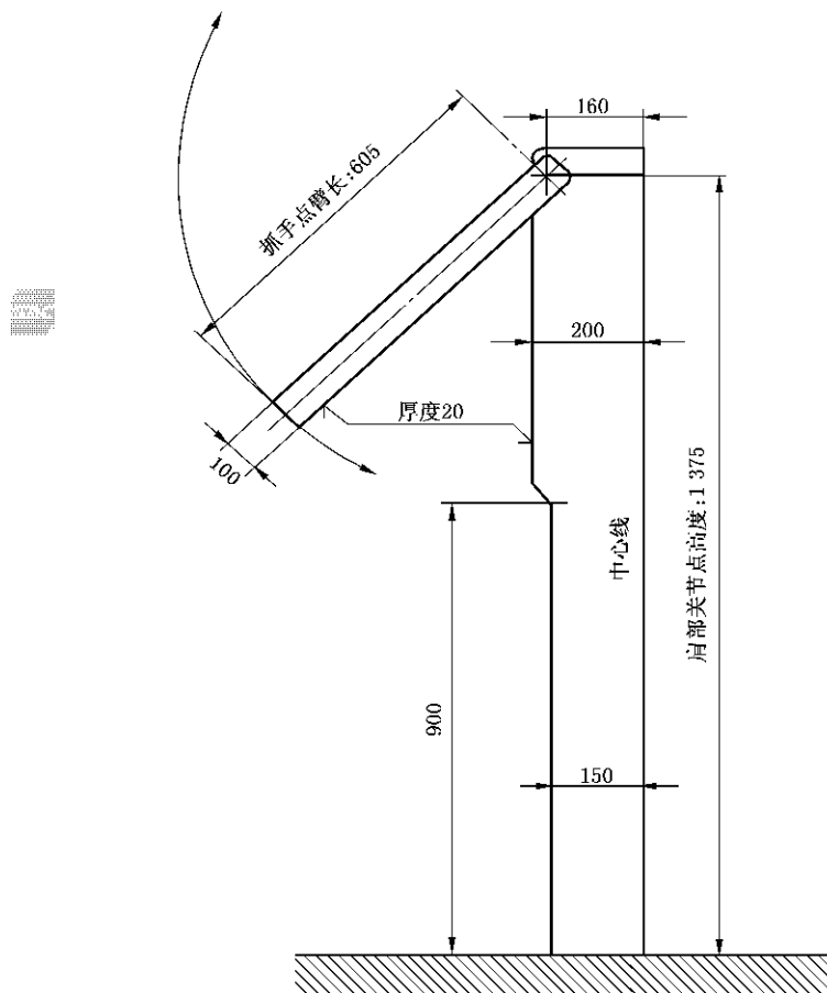
图 18 模拟站立乘客的测量装置
